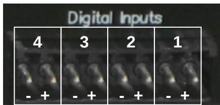
Abbildung 6 - Digitale Eingänge
